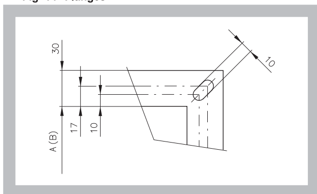
Fig. 14 Flanges
