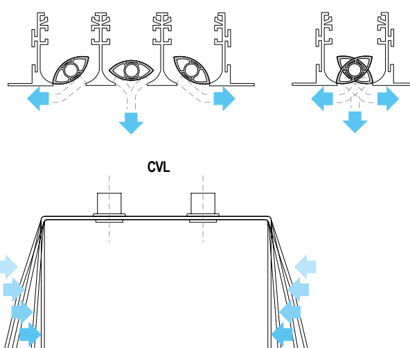
Modifica configurazione CVL da PDL 3 a PDL 2 con pressione delle dita Configuration change CVL to PDL 3 to PDL 2 with finger pressure
