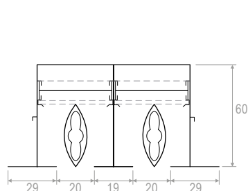
DLN250 2 feritoie - slots
