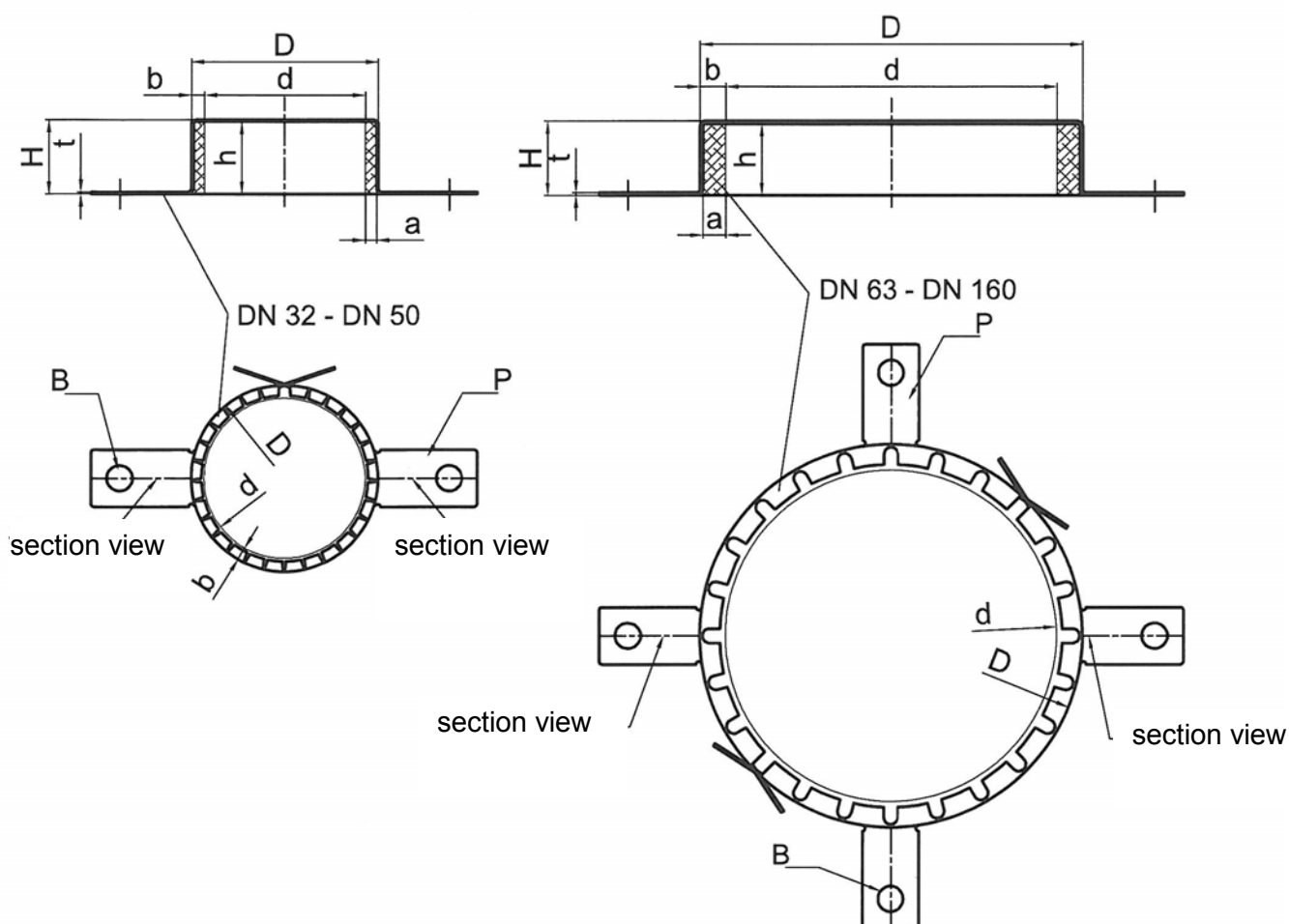
pipe collar "BIS Pacifyre® AWM III"
