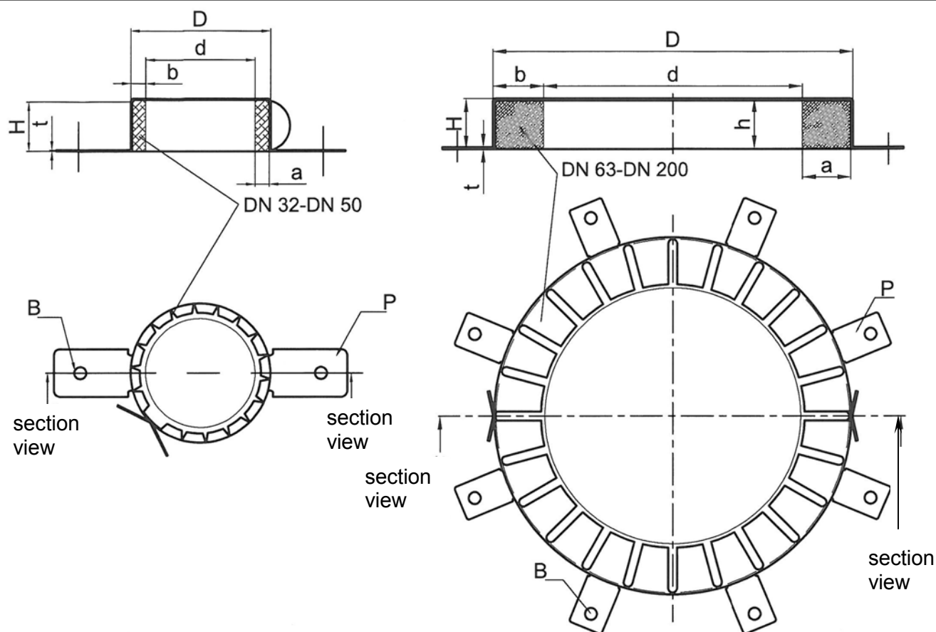
pipe collar "BIS Pacifyre® AWM II"
